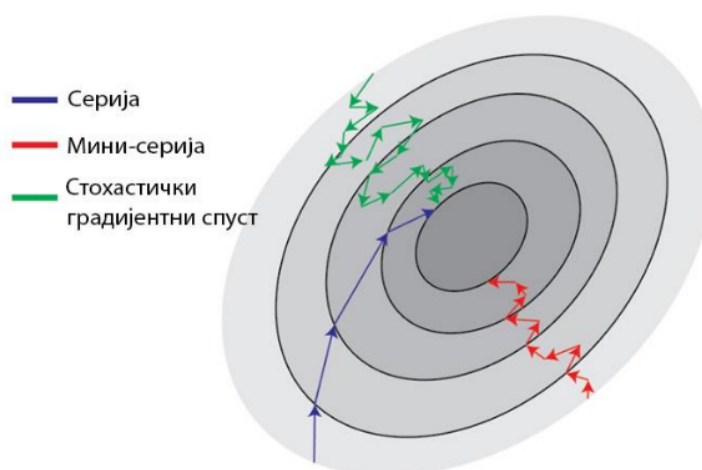
Слика 2-17: Поређење оптимизације функције губитка за читаву серију (плава путања), мини-серија (црвена путања) и стохастички градијентни спуст (зелена путања) [110]
