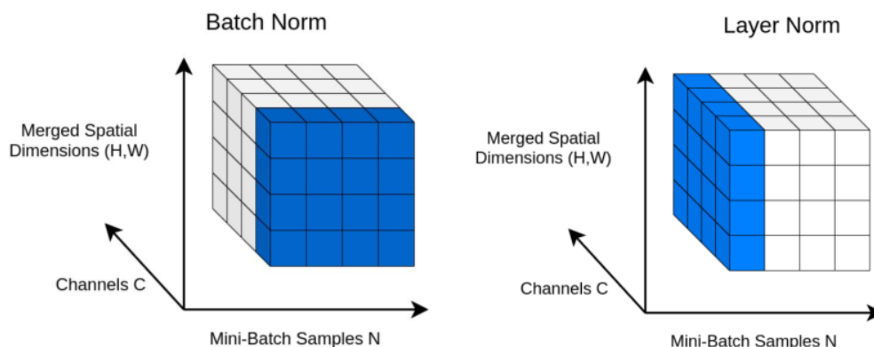
Слика 2-13: Поређење нормализације на нивоу серије и на нивоу слоја [57], [106], [107]
