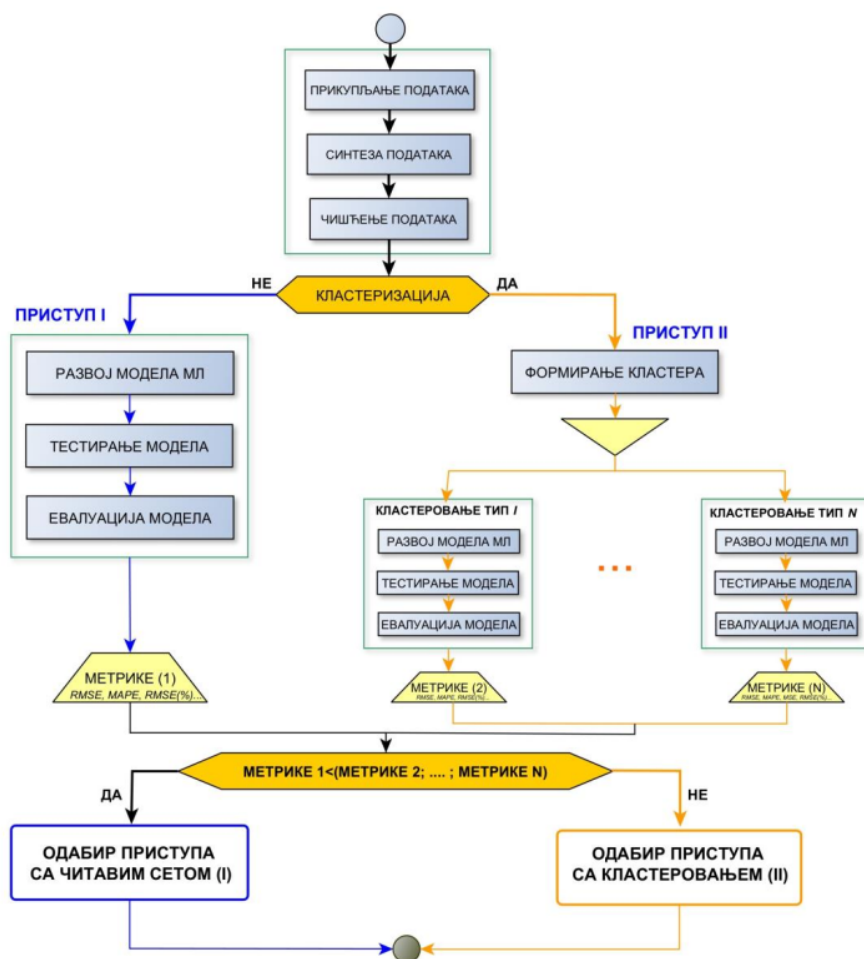
Слика 3-4: Дијаграм тока истраживања
