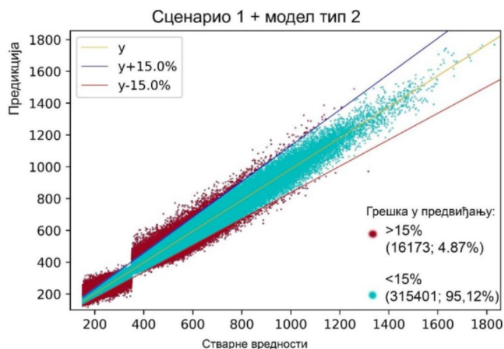
Слика 4-32: Распореда предикција добијена комбинацијом првог сценарија и модела типа 2
