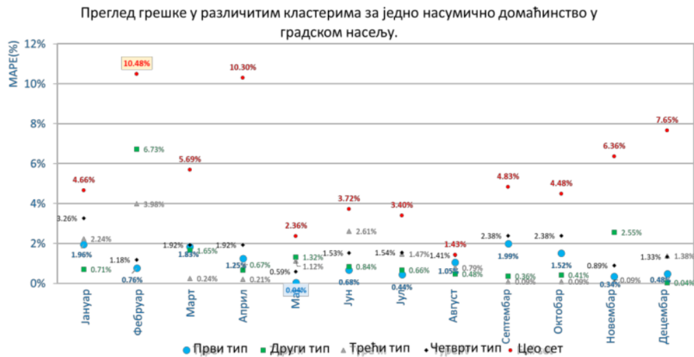
Слика 4-48: Средње вредности MAPE(%) за једног насумичног потрошача, добијене помоћу модела типа B , за сваки тип кластеровања и скуп у целости [54]
