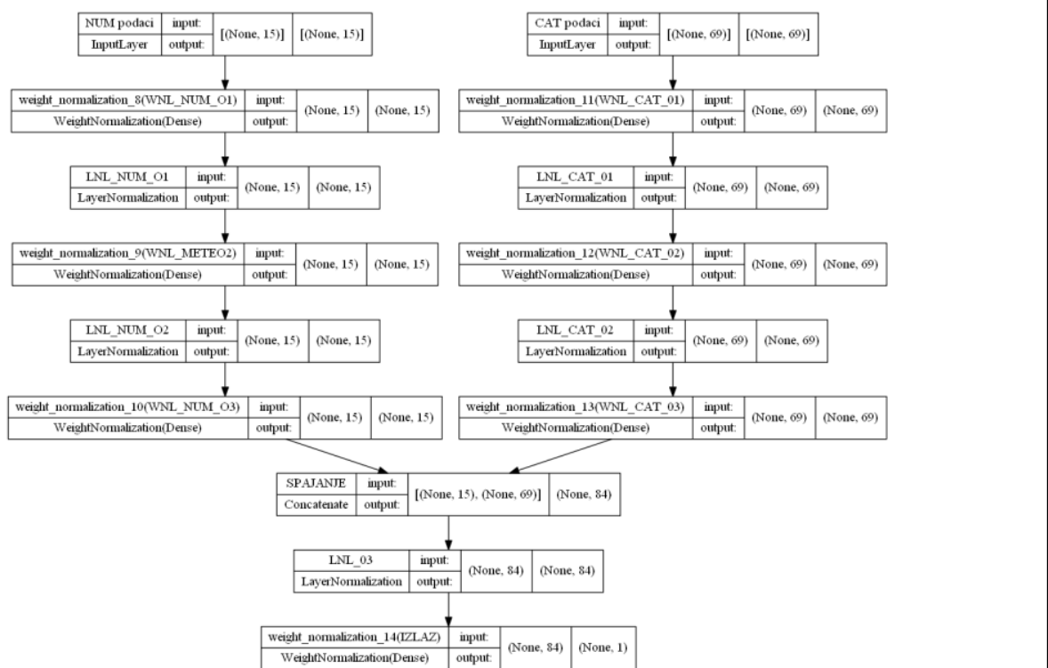
Слика 6-8: Програмска штампа (шема) архитектуре модела са две улазне гране нумеричких и категоријских обележја
