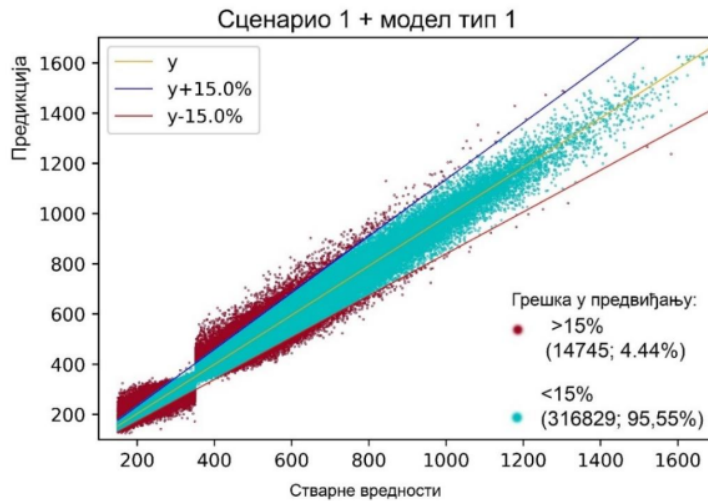
Слика 4-31: Распореда предикција добијена комбинацијом првог сценарија и модела типа 1
