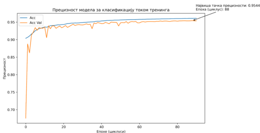
Слика 4-57: Дијаграм прецизности модела на тренинг и валидационом скупу
