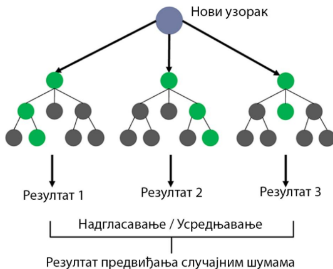
Слика 2-6: Приказ структуре случајне шуме [77]
