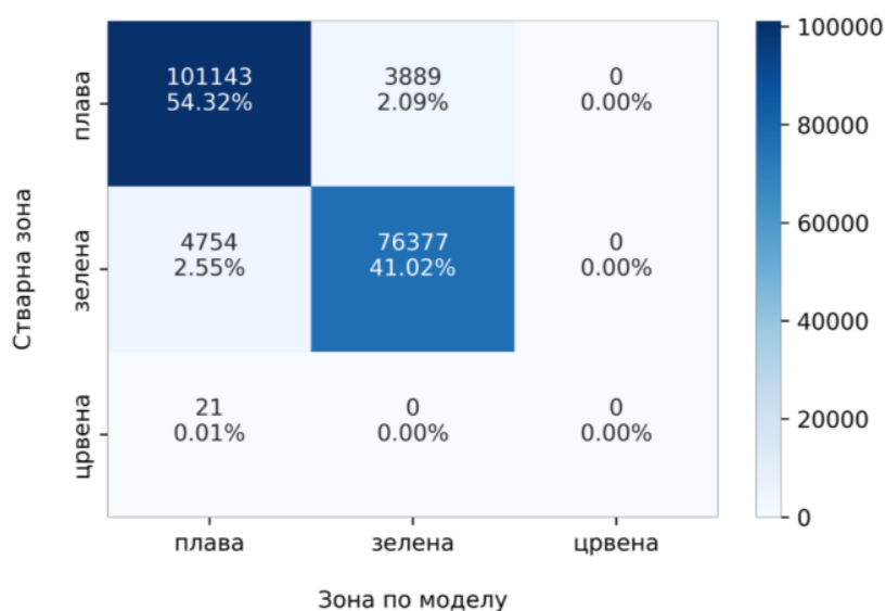
Слика 4-59: Матрица конфузије за предвиђање зоне потрошње
