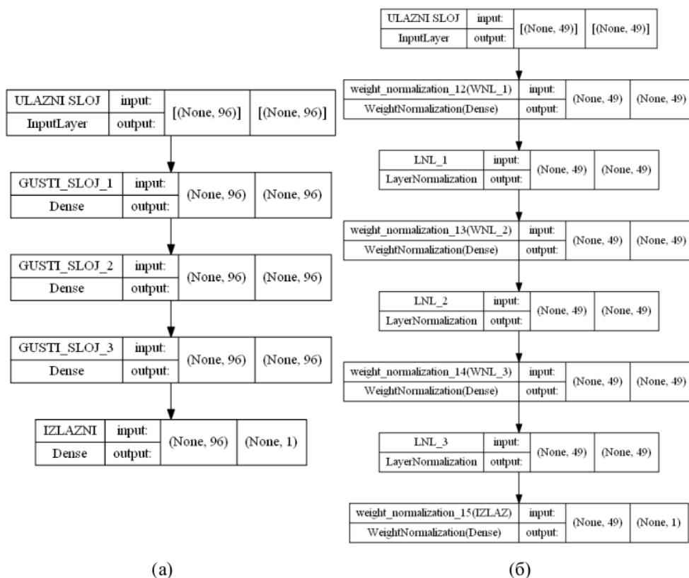
Слика 4-41: Модел А (а) и модел Б (б) - структура слојева
