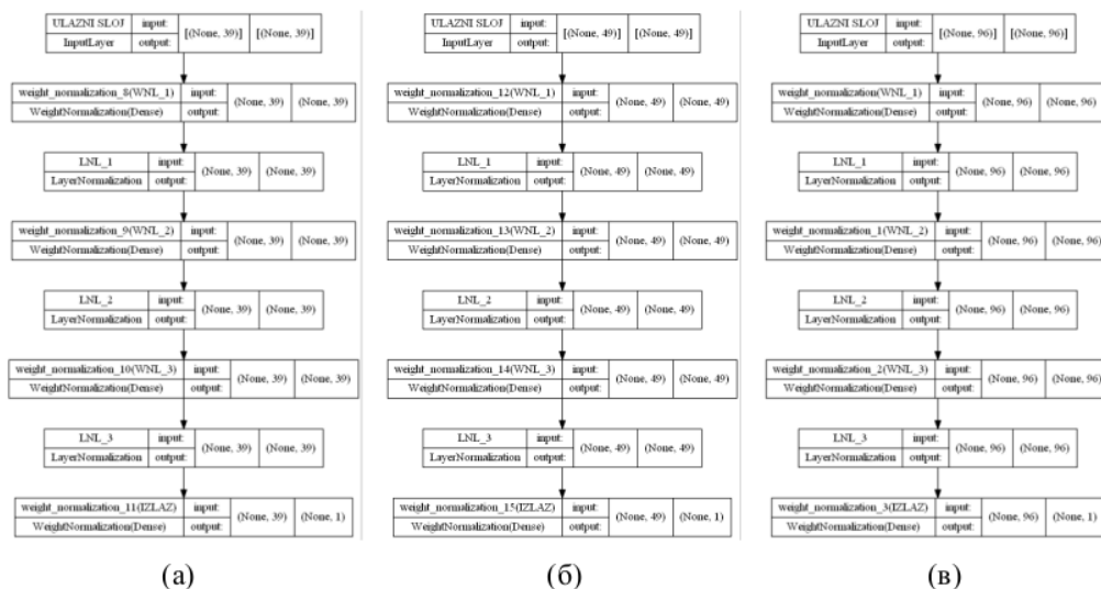
Слика 4-40: Модел за кластер једног месеца (а), кластер једног годишњег доба (б) и за скуп у целисти (в) – модел Б
