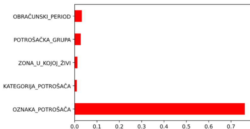
Слика 4-5: Важност обележја у иницијалном скупу података
