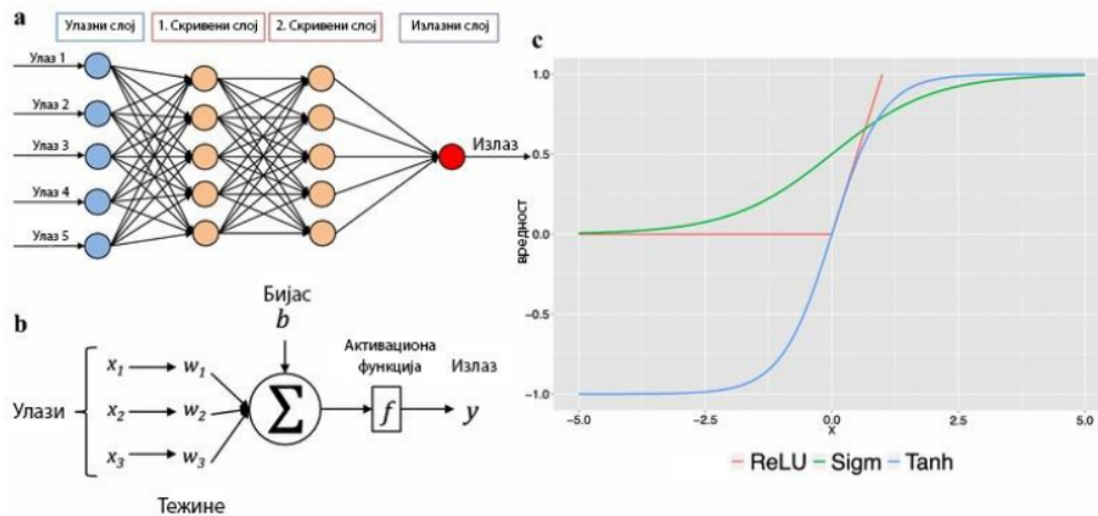
Слика 2-14: Активационе функције [105]
