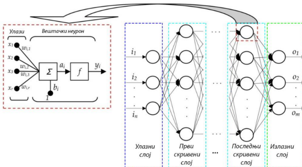
Слика 2-11: Општи приказ структуре потпуно повезане ANN [63]
