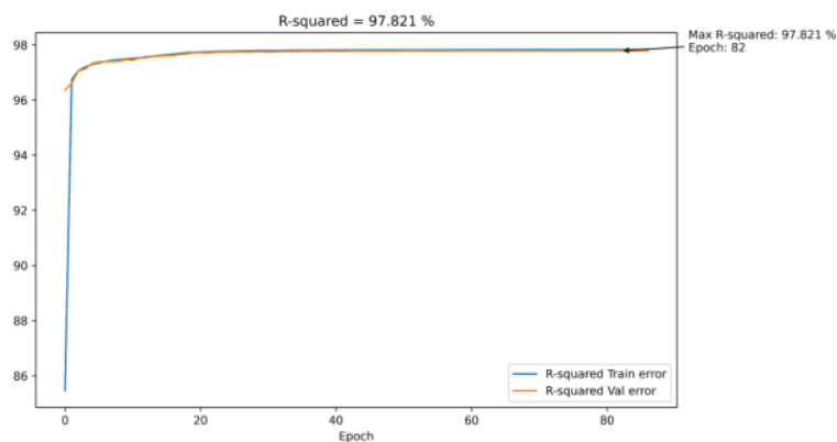
Слика 6-9: Коefицијент детерминације ( R^2 ) за модел са две улазне гране (нумеричких и категоријских обележја)
