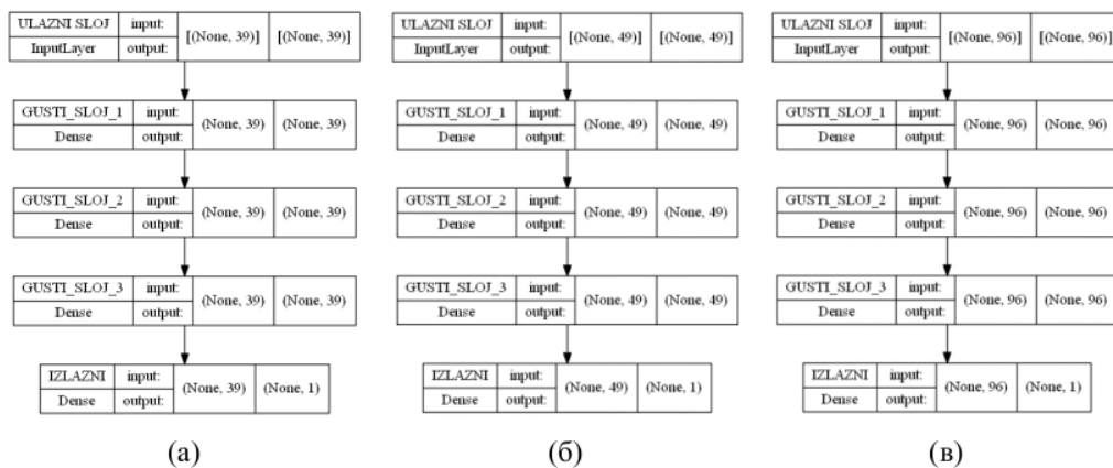
Слика 4-39: Модел за кластер једног месеца (а), кластер једног годишњег доба (б) и за скуп у целисти (в) – модел А
