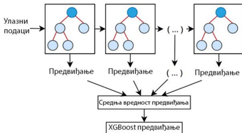
Слика 2-7: Приказ структуре екстремног градијентног буста [79]
