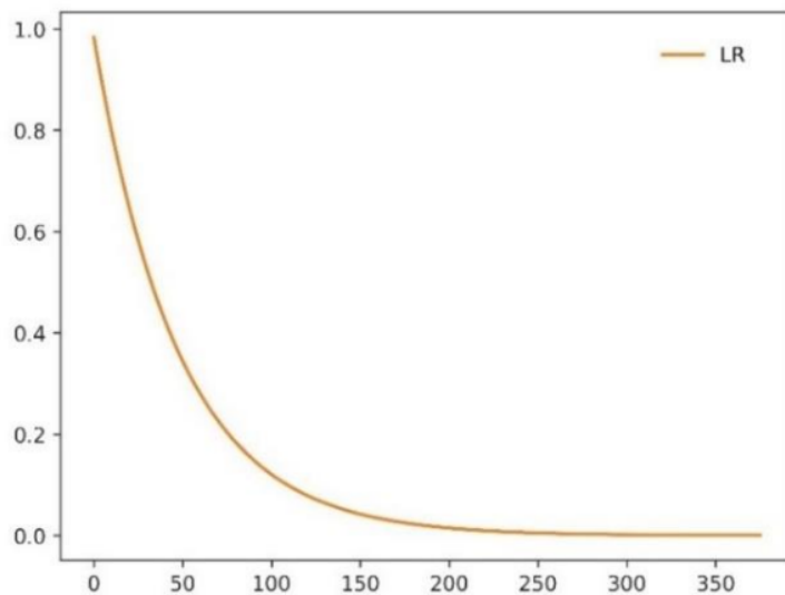
Слика 4-23: Промена стопе учења током епоха
