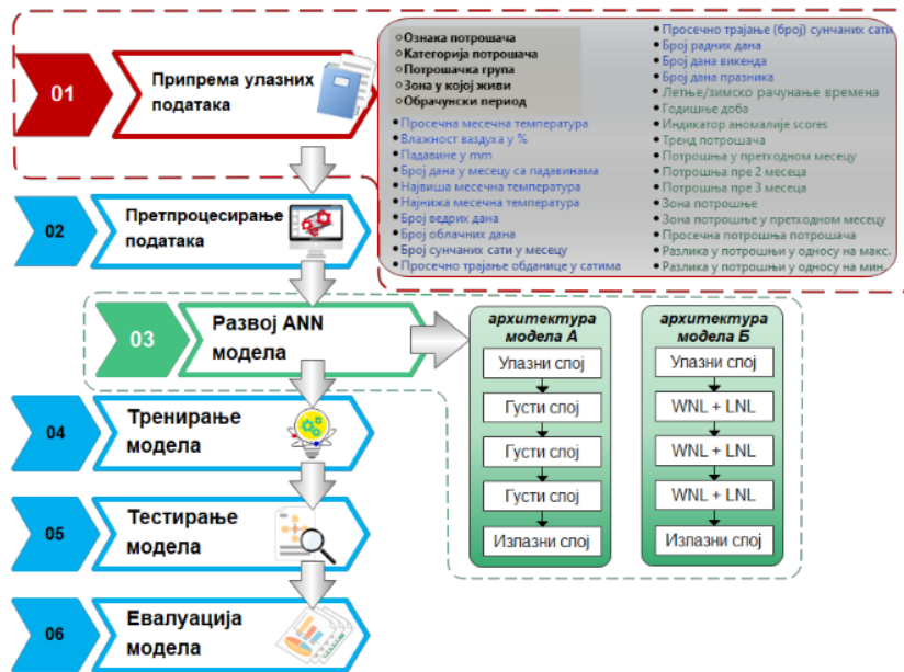
Слика 4-36: Дијаграм тока активности у изради и оцени модела по фазама (према методологији представљеној у 3.3.1, Слика 3-3) [54]
