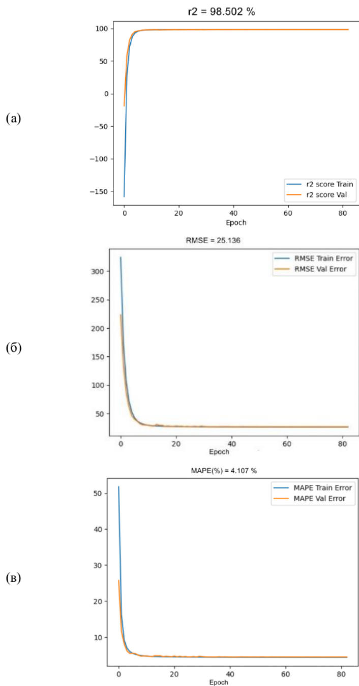
Слика 4-27: Коefицијент детерминације (а), корен средње квадратне грешке (б) и средња просечна апсолутна грешка (в) за сценарио 2 + модел типа 1 (модел са 85 неурона)
