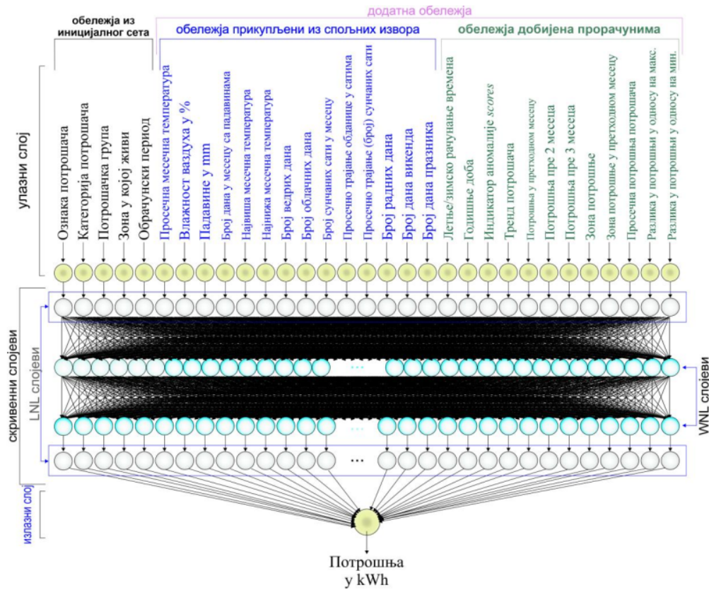
Слика 4-26: Архитектура предложеног модела (тип 1) [144]
