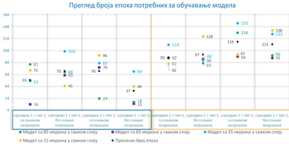
Слика 4-30: Број епоха за сваки од сценарија/модела/типова кодирања и броја неурона у мрежи [144]
