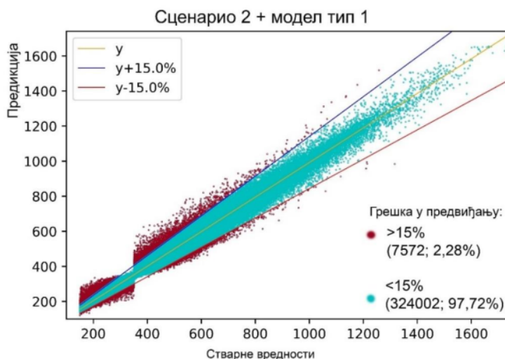
Слика 4-33: Распореда предикција добијена комбинацијом другог сценарија и модела типа 1
