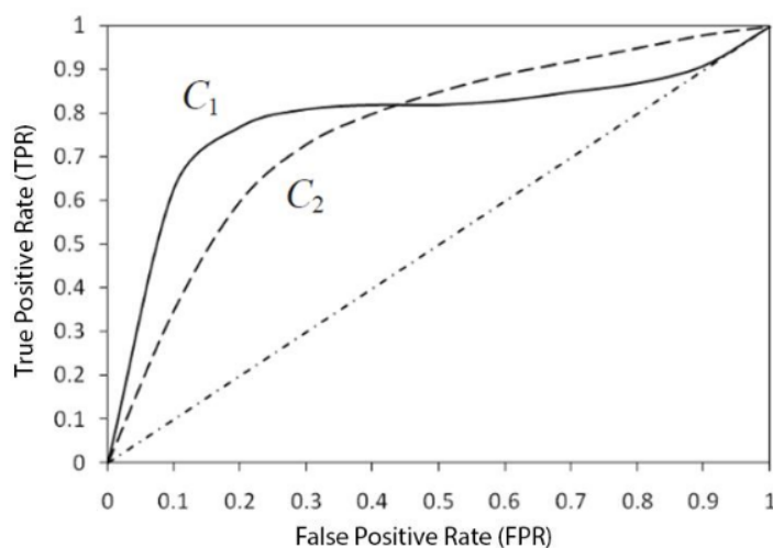
Слика 2-3: ROC крива за два класификатора [69]
